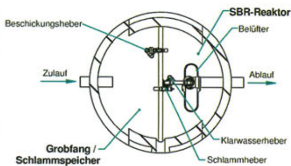
B-B
