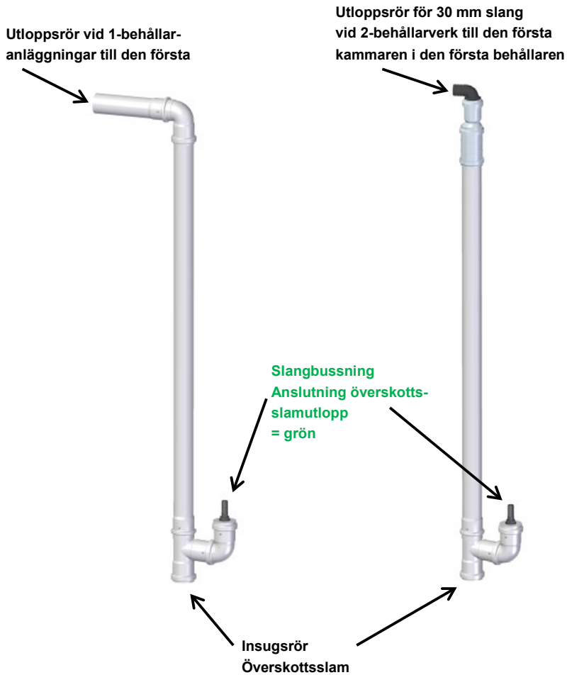
Figur 4: Hävert för överskottsslam
