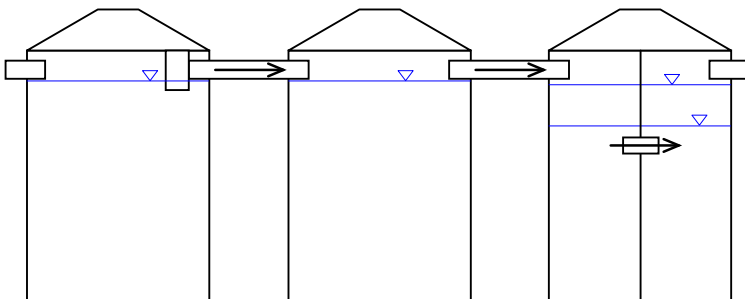
Figur 16: 3-behållaranläggning utan undervattensförbindning
