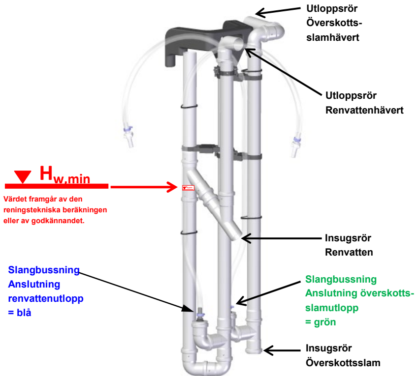
Figur 6: Hävertar för renvatten och överskottsslam som enhet
