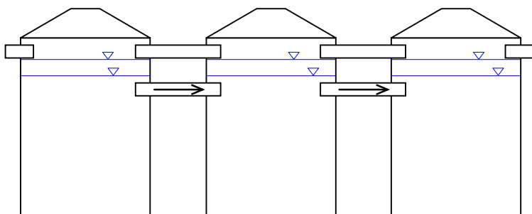
Figur 13: 3-behållaranläggning med undervattensförbindning
