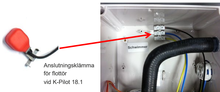
Figur 27: Anslutning flottörställare i K-Pilot 18.1
