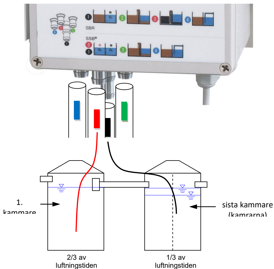
Figur 9: Slanganslutningar på styrningen
