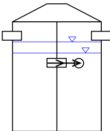
Figur 11: 3-kammarschakt (1 behållare) med undervattensförbindning
