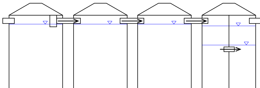
Figur 17: 4-behållaranläggning utan undervattensförbindning
