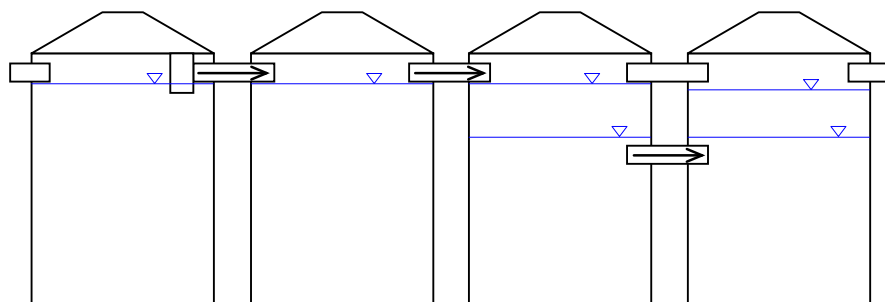
Figur 18: 4-behållaranläggning, främre behållare utan undervattensförbindning
