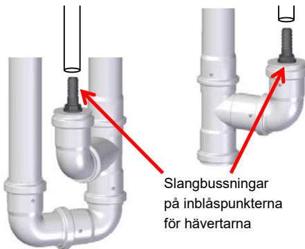
Figur 8: Fastsättning av slangar på hävert och placering i behållaren
