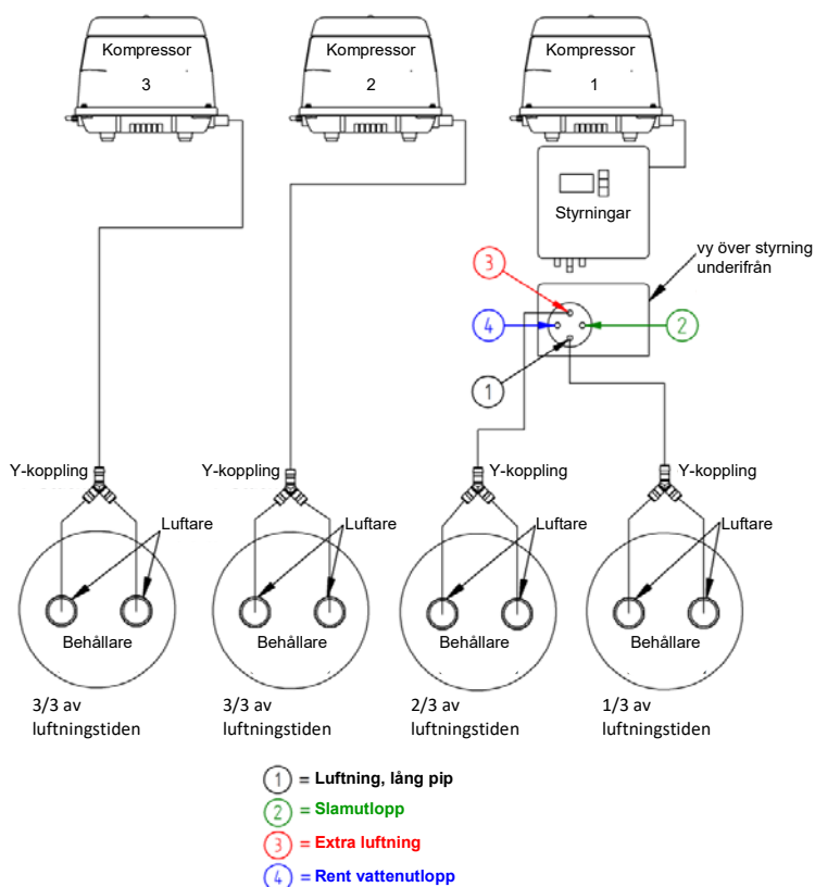
Figur 24: 3-kompressoranläggning i 4 behållare
