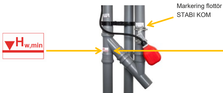
Figur 26: Fastsättning av flottörställare
