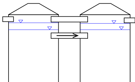
Figur 12: 2-behållaranläggning med undervattensförbindning
