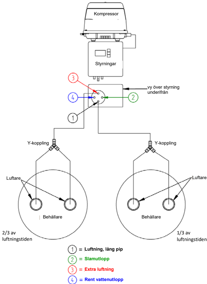
Figur 21: 2-behållaranläggning
