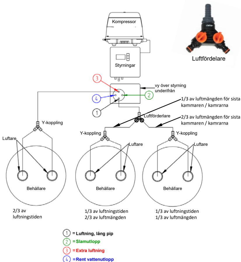
Figur 22: 3-behållaranläggning
