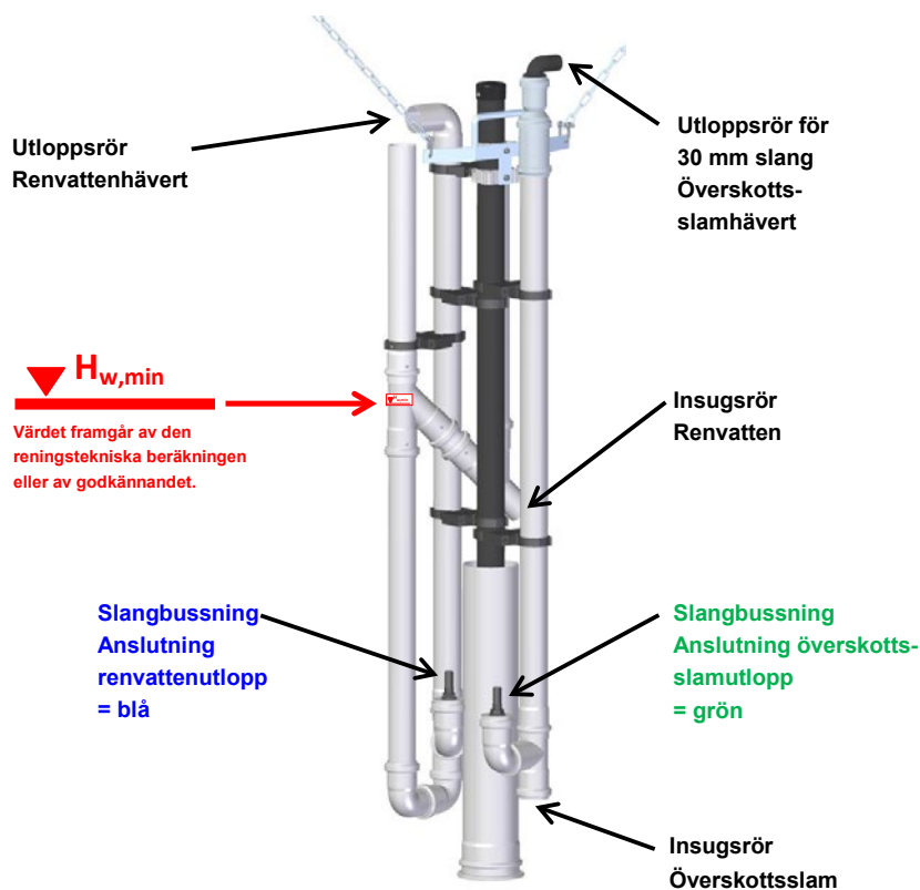
Figur 5: Renvatten- och överskottsslamhävert i kedja
