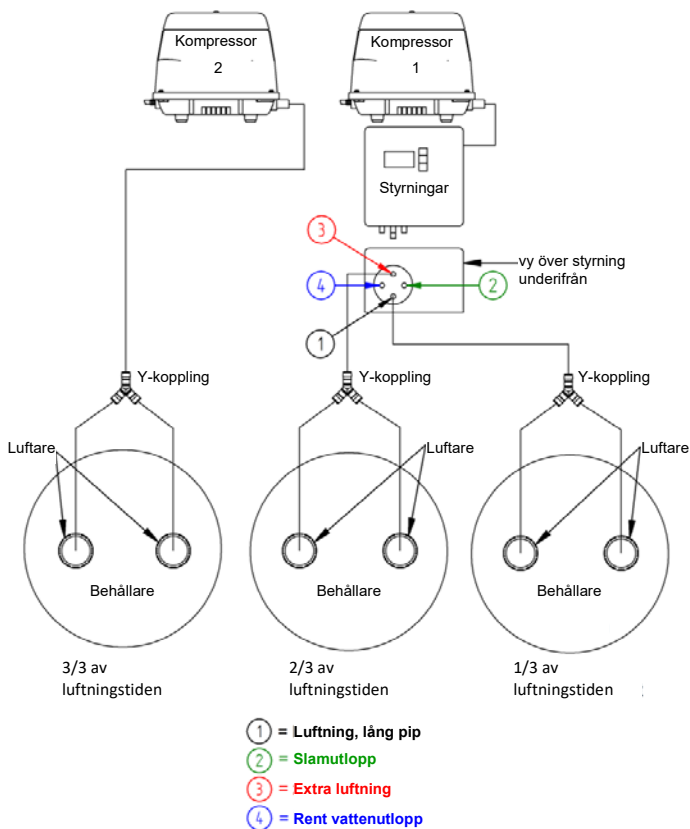
Figur 23: 2-kompressoranläggning i 3 behållare
