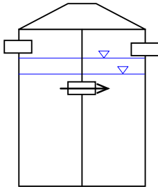
Figur 10: 2-kammarschakt (1 behållare) med undervattensförbindning
