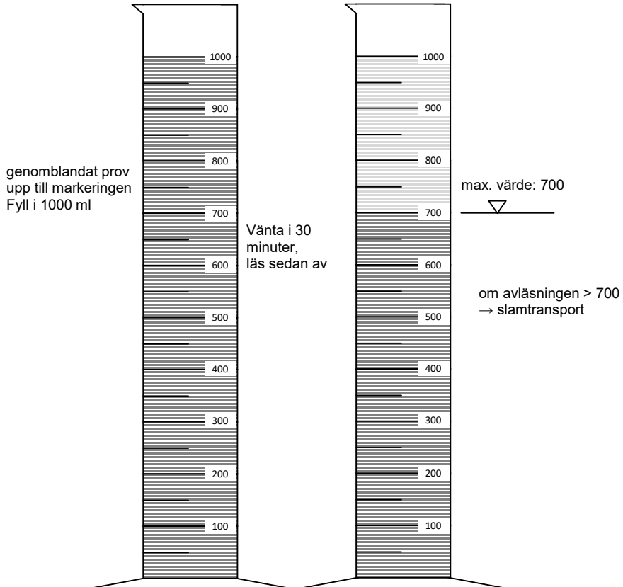
Figur 31: Mätning av slamvolym
