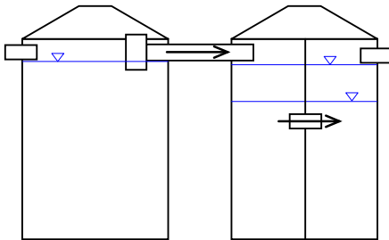
Figur 15: 2-behållaranläggning utan undervattensförbindning
