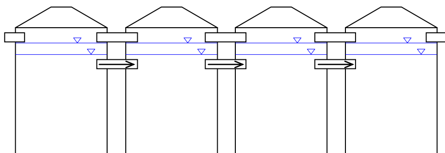
Figur 14: 4-behållaranläggning med undervattensförbindning
