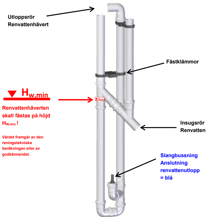
Figur 3: Renvattenhävert
