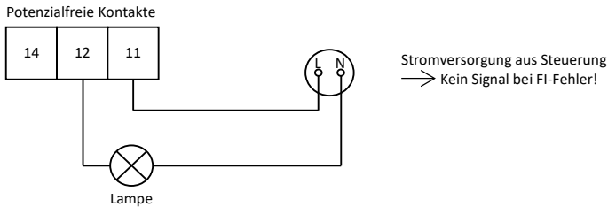
Abbildung 12: Potenzialfreier Kontakt mit Fehlermeldung – Stromversorgung aus der Steuerung
