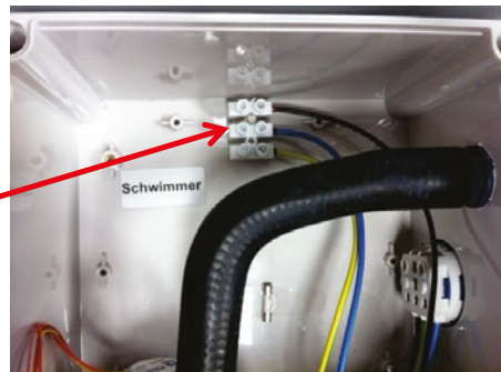
Abbildung 14: Anschluss Schwimmerschalter bei Steuerungs-Typ K-Pilot 18.1
