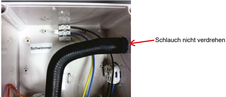
Abbildung 3: Der Schlauch im Inneren der Steuerung darf nicht verdreht werden.
