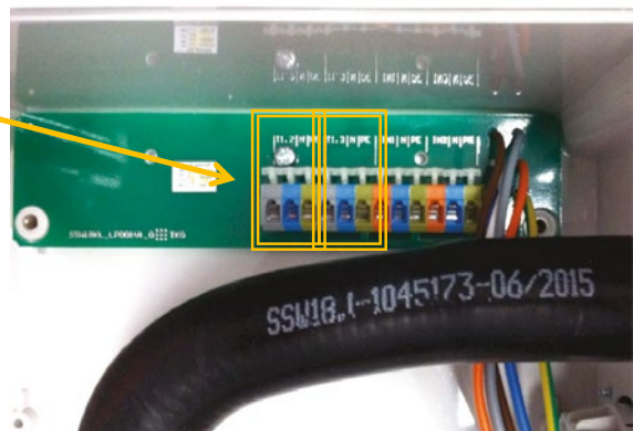
Abbildung 22: Anschluss Klarwasserpumpe in Steuerung K-Pilot 18.3
