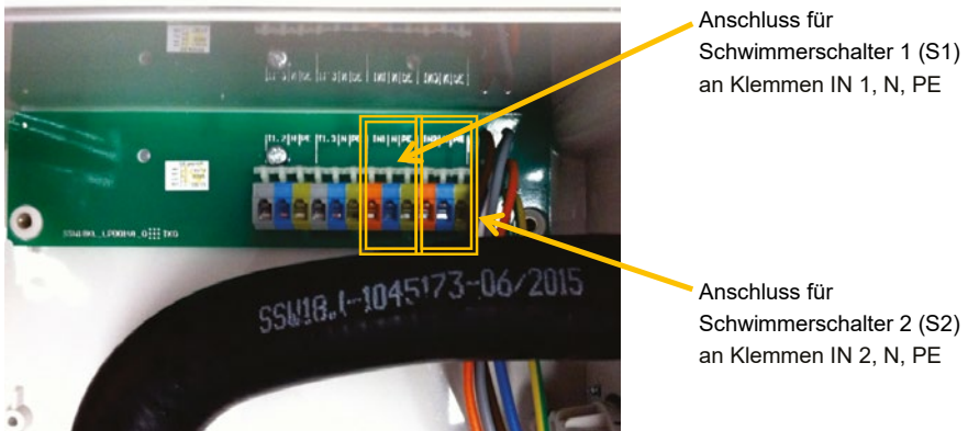
Abbildung 20: Anschluss Doppel-Schwimmerschalter bei Steuerung K-Pilot 18.3
