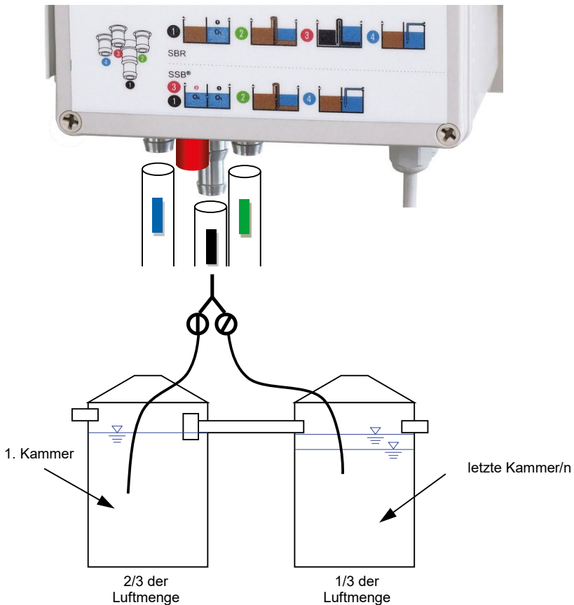
Abbildung 8: Schlauchanschlüsse – Belegung bei SSB-Sondervariante
