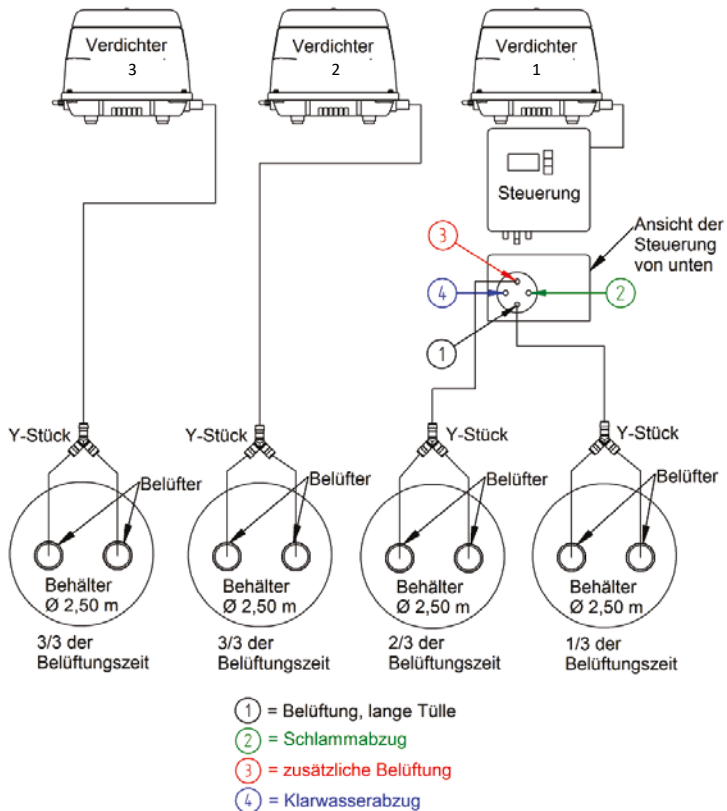
Abbildung 7: Schlauchanschlüsse – Belegung bei SSB-3-Verdichter-Anlage (4 Behälter)
