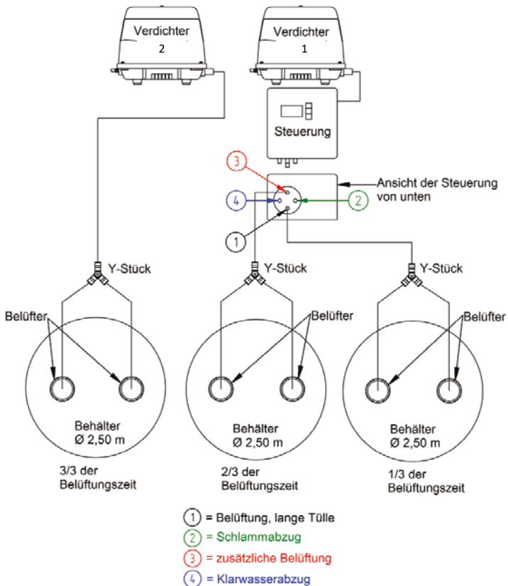
Abbildung 6: Schlauchanschlüsse – Belegung bei SSB-2-Verdichter-Anlage (3 Behälter)
