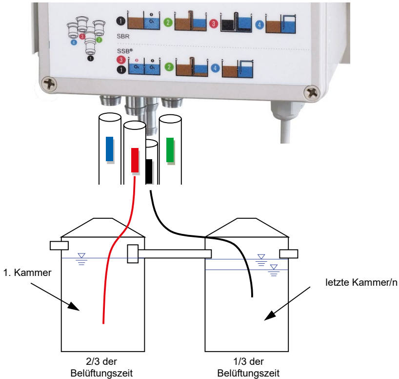
Abbildung 5: Schlauchanschlüsse – Belegung bei SSB-Standardvariante
