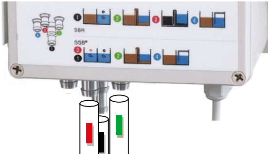
Abbildung 10: Steuerung mit FB und WSB-Luftschlauchanschlüssen
