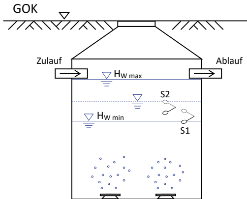
Abbildung 35: Anlage mit Doppelschwimmerschalter
