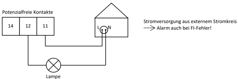
Abbildung 13: Potenzialfreier Kontakt mit Fehlermeldung auch bei Stromausfall
